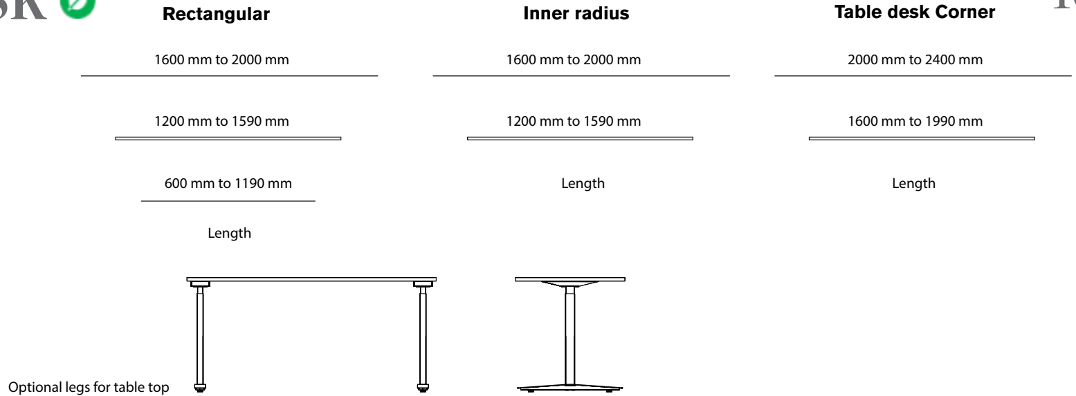
Optional legs for table top
