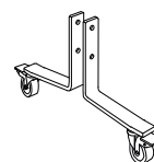
Fotvinkel med läsbara hjul l x b x h 190 x 40 x 122 mm
