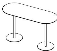
ODETTE TABLE (OD - 63) Top SC-08 W:175 D:70 Base SC-116+SC-116 H:100
