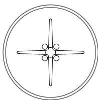
Ø 1250 H 730/900
