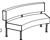
SA2250 H 780 SH 450 B 1470/1960/2450 D 600
