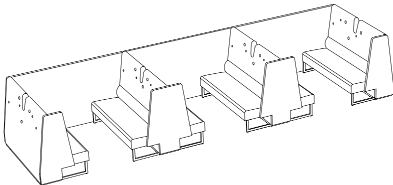
SA300 rak rygg (1) x4 SA310 låg rak sits (5) x4 SA350 kupévägg mellan (17) x1
