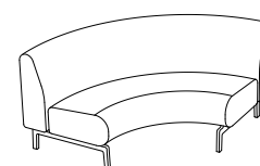
SA410 sväng soffa 90° R 600, bengavel x2 H 800/830 SH 440/470 B 1300 D 1300
