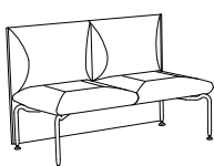
SA820 fristående (6) H 850 SH 450 B 1280 D 650
