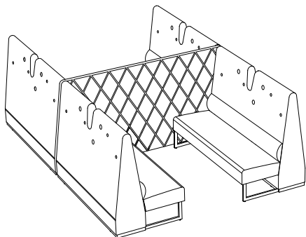
SA300 rak rygg (1) x4 SA310 låg rak sits (5) x4 SA350 kupévägg mellan (17) x1
