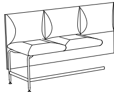
SA820 hörnkoppling (11) H 1030 SH 630 B 1910 D 650
