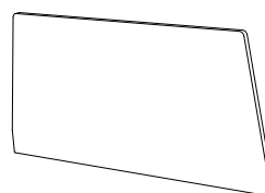
SA350 kupévägg/mellan (17) H 1315 B 2620 D 45
