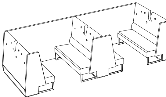
SA300 rak rygg väggställd (3) x1 rak rygg (1) x2 SA310 låg rak sits (5) x4 SA350 kupévägg vänster (19) x1 kupévägg rak (18) x1 SA320 gavel enkel (11) x1 gavel dubbel (12) x1 gavel väggställd (13) x1
