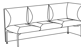
SA830 fristående (18) H 850 SH 450 B 1295 D 665
