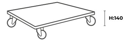
HJULSATS
