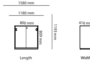
Sliding door
